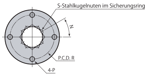
CPS-E03~10T Sicherungsring (Typ E) CPS-L03T Sicherungsring (Typ L)
