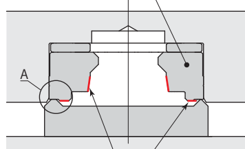
Sicherungsring Typen CPS-D□, CPS-E□, CPS-L□
